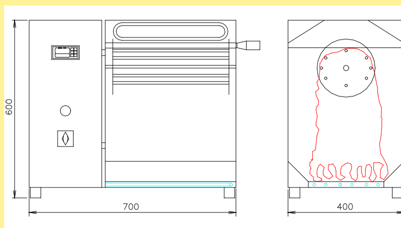
vista frontal y lateral de BAC-400mm
